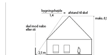
Illustration af det skrå højdegrænseplan jf. § 5.4
