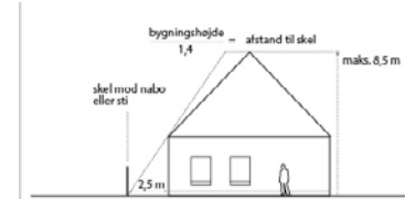
højdegrænseplan jfr. § 5.4
